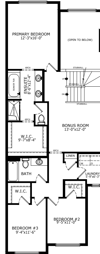
UPPER: 1160 SQ FT
